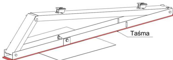
Sposób zabezpieczenia krawędzi w przypadku membrany starszej niż 5 lat
