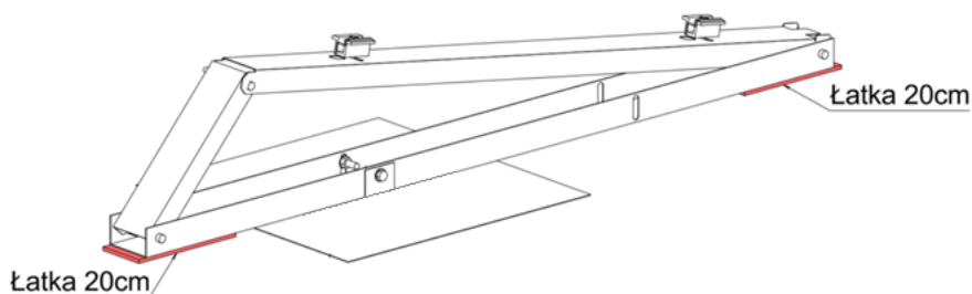
Sposób zabezpieczenia krawędzi w przypadku membrany młodszej niż 5 lat
