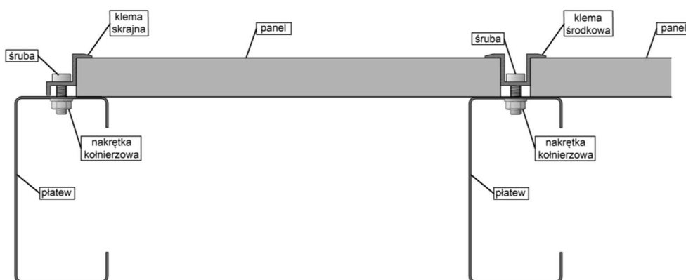
Rys. Schemat poglądowy montażu modułów
