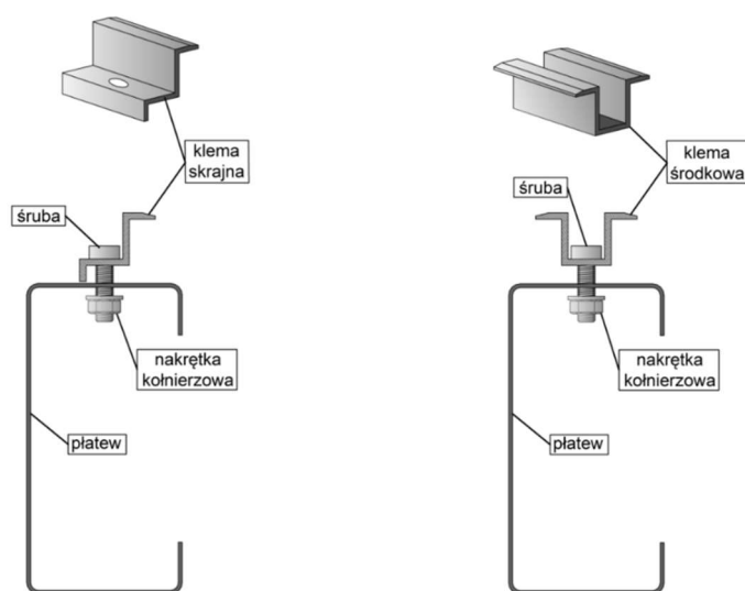
Rys. Schemat poglądowy wstępnego montażu klem
